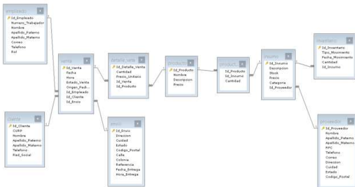
Figura 5. 12 Moedelo relacional
