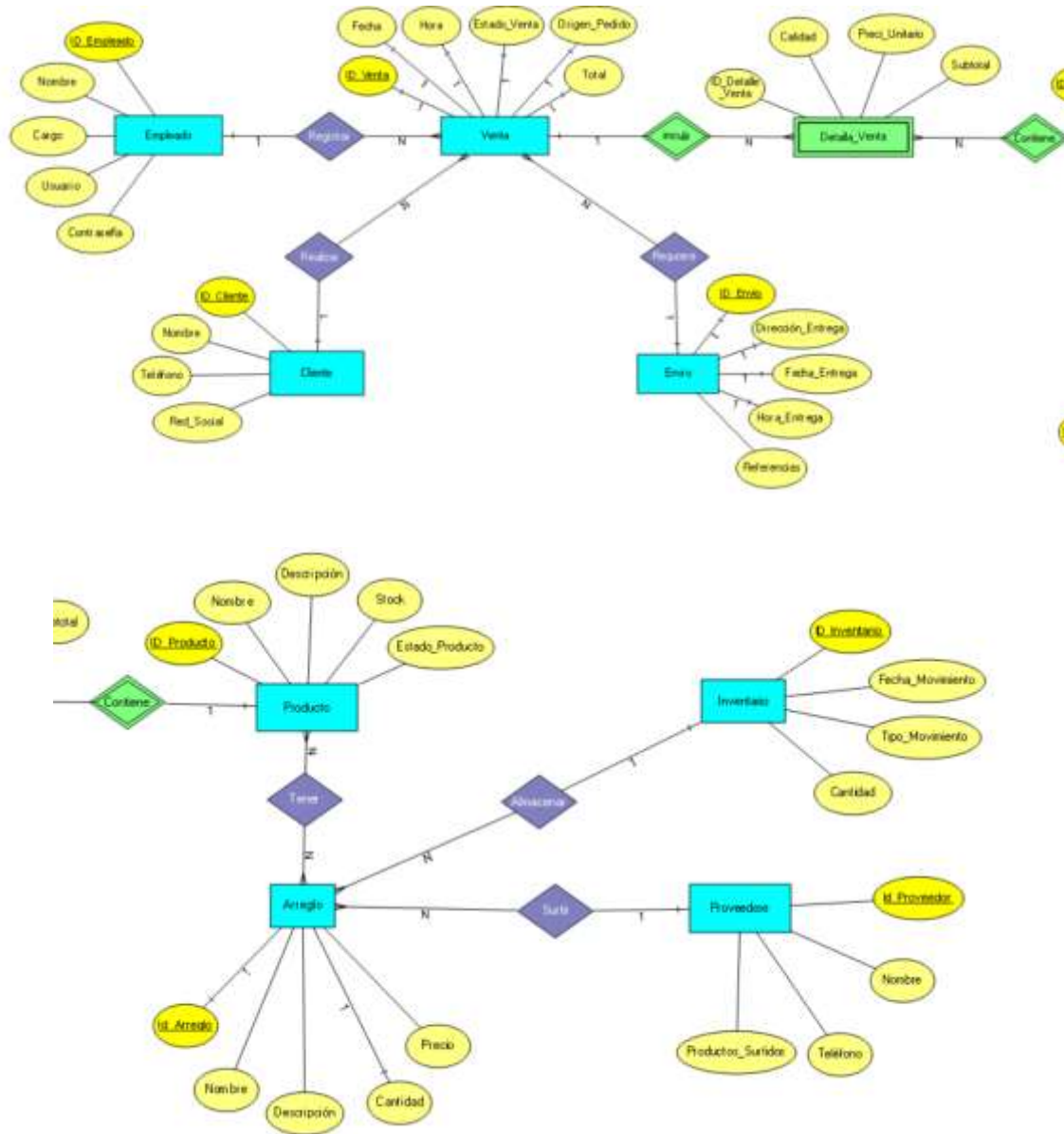
Figura 5. 11 Modelo entidad-relación
