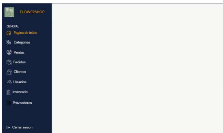
Figura 5. 33 Pantalla inicio
